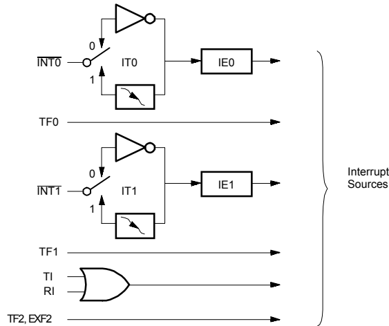
图 20 中断源
