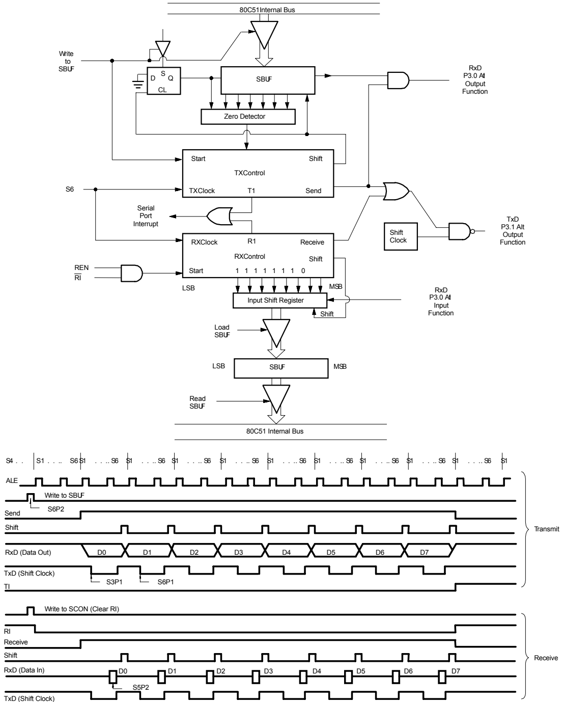
图 14 串口模式 0
