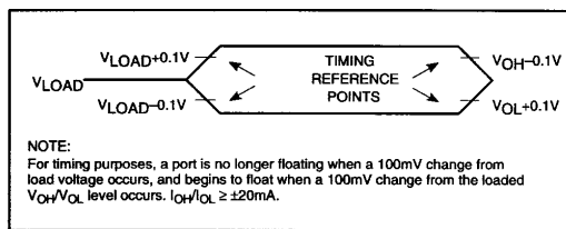
图 32 悬浮波形
